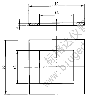
图4 拉伸用垫板
