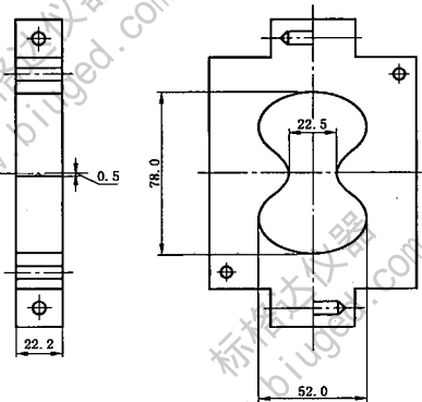
图 7 “8”字形金属模具
