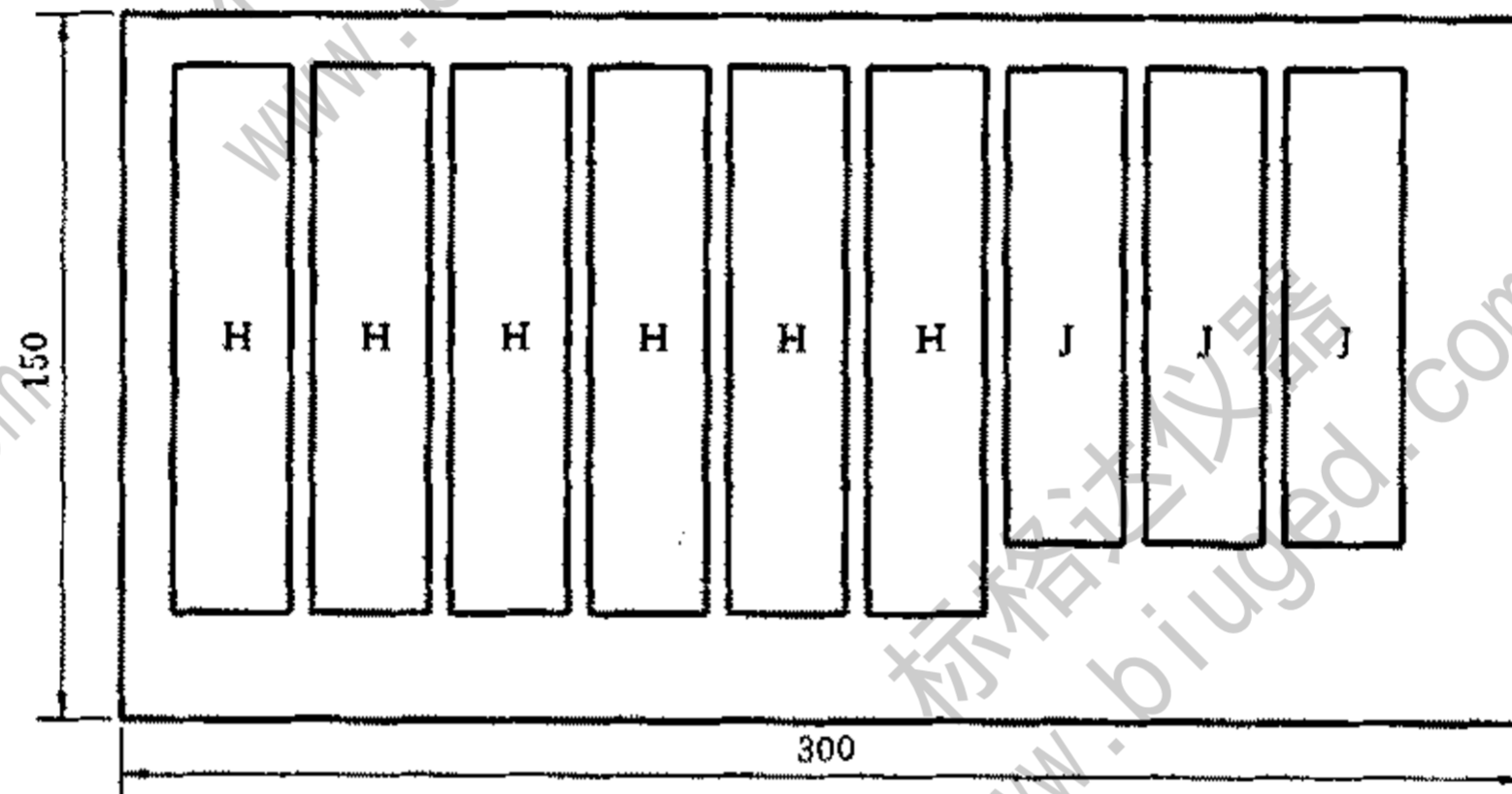
图 3 防水涂料的取样图
