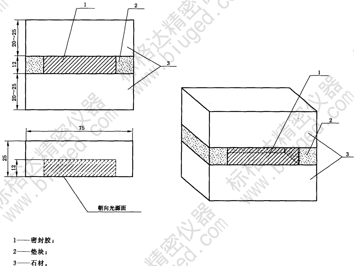
图 1 试件形状
