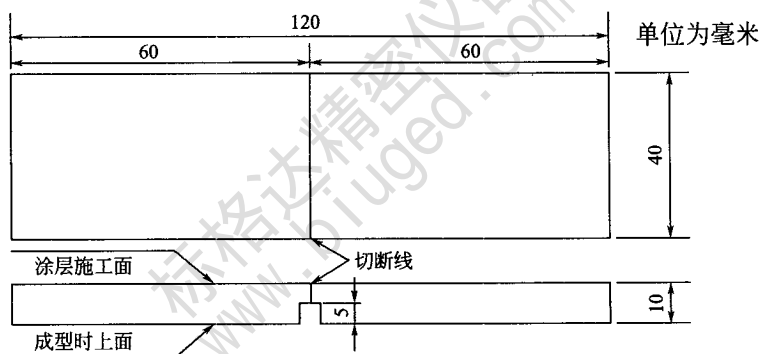
图 A.1 基材形状
